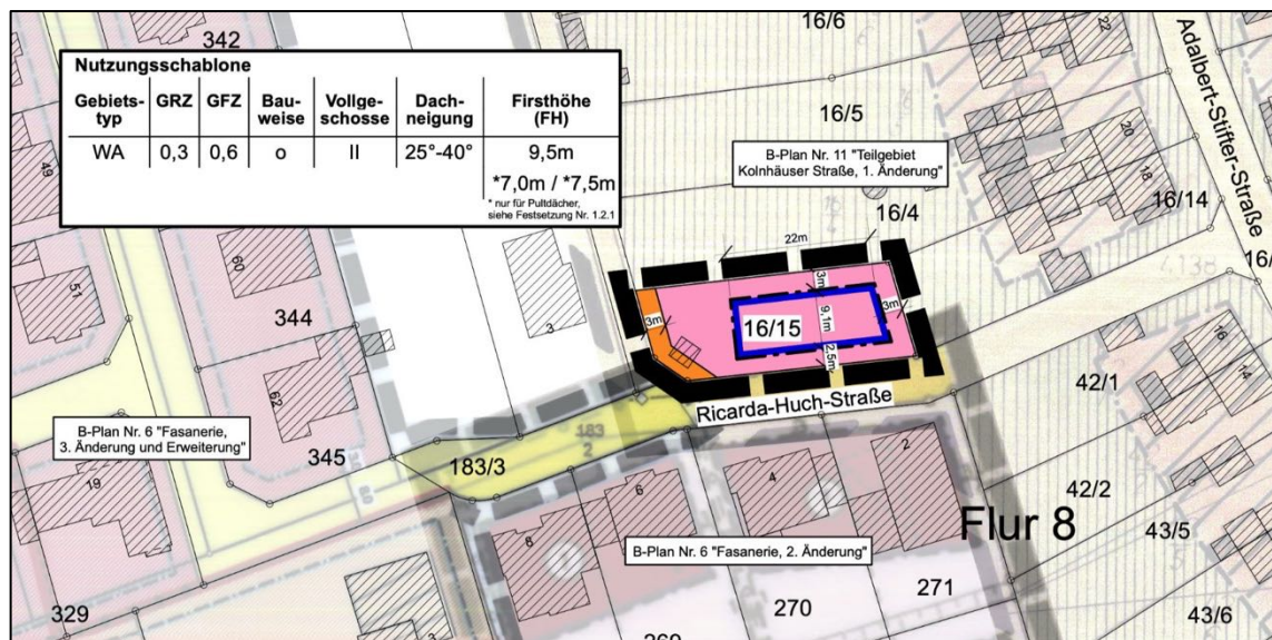
Abbildung 14: Bebauungsplan – Planteil
