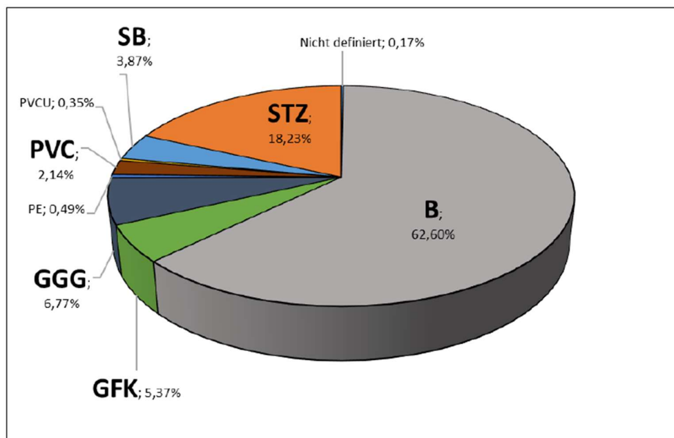
Abbildung 2: Verteilung der Werkstoffe bei den Verbandskanälen
