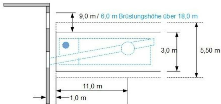
Bild: Aufstellfläche rechtwinklig zur Außenwand
