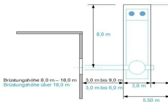
Bild: Aufstellfläche entlang der Außenwand
