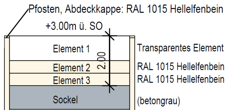
Abb. 4 Aufbau Lärmschutzwandsegment
