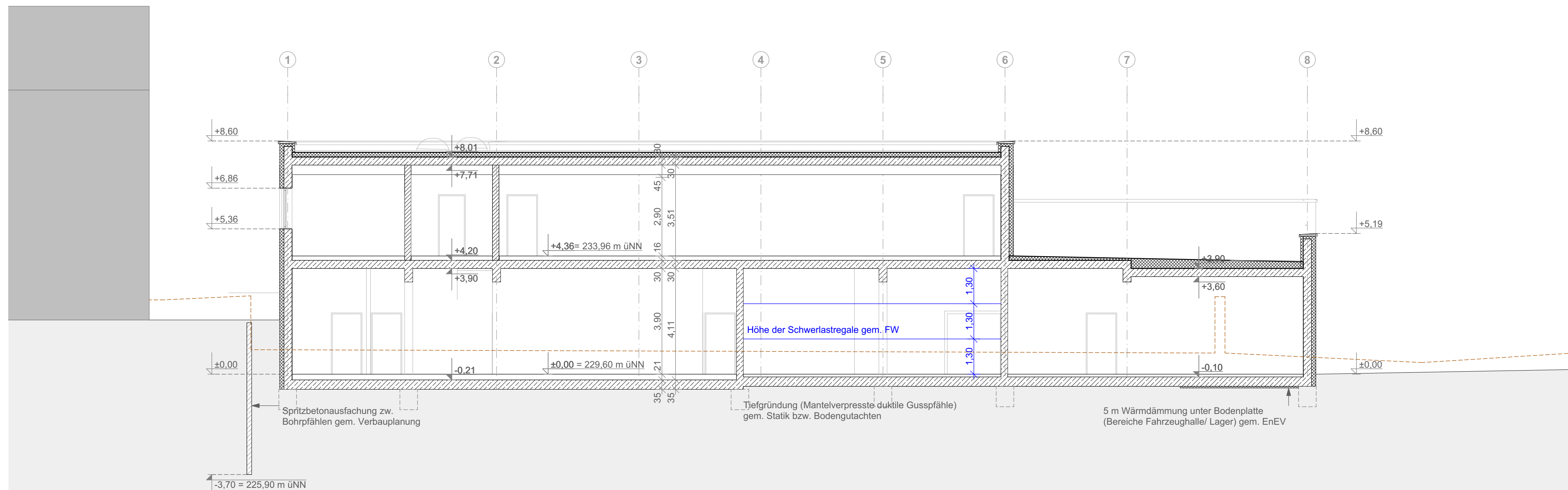
Schnitt C-C
